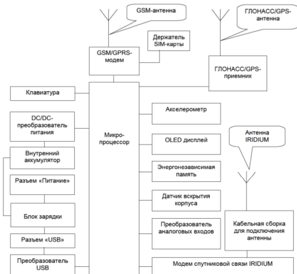
Рисунок 2. Структурная схема устройства
